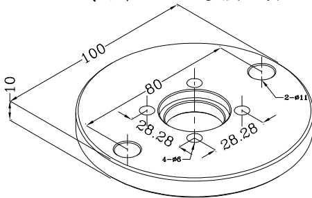
专用法兰连接底板
