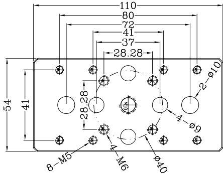
底部安装孔位图
