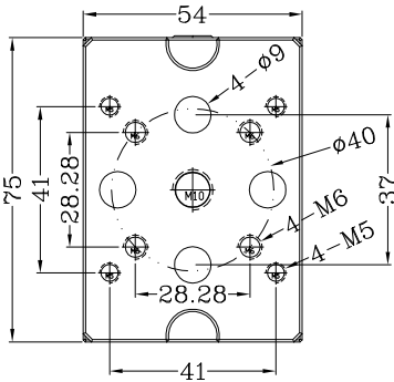
底部安装孔位图
