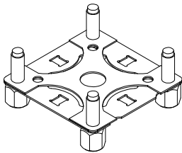
专用法兰连接底板
