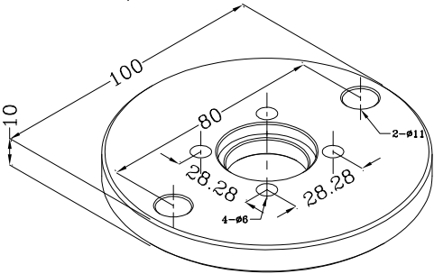
专用法兰连接底板
